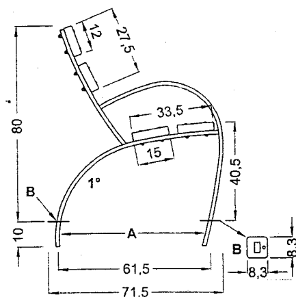
Fianco - sostegni Sx-Dx
