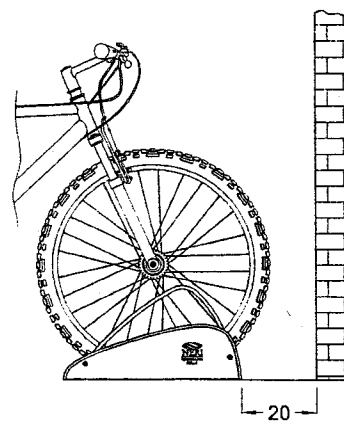
Fianco Distanza dalla parete (*) Scala 1:20
