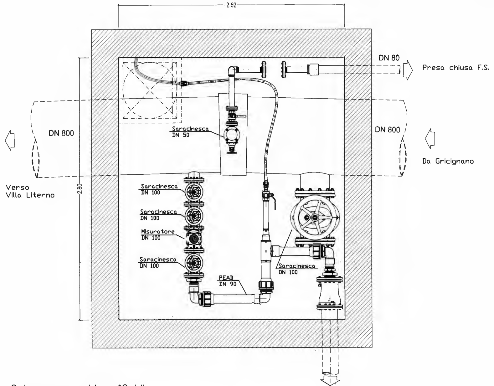
Schema pozzetto n°3 Via larga Carinara 40.989907, 14.232814
